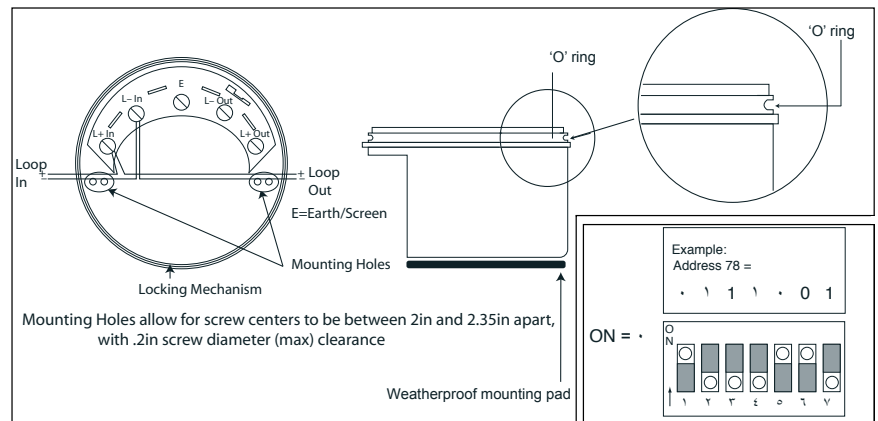
Fig 1. Wiring diagram
